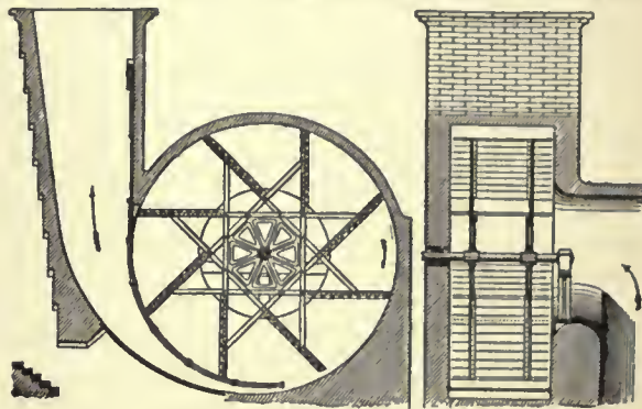
FIG. 12.—Guibal Fan.
